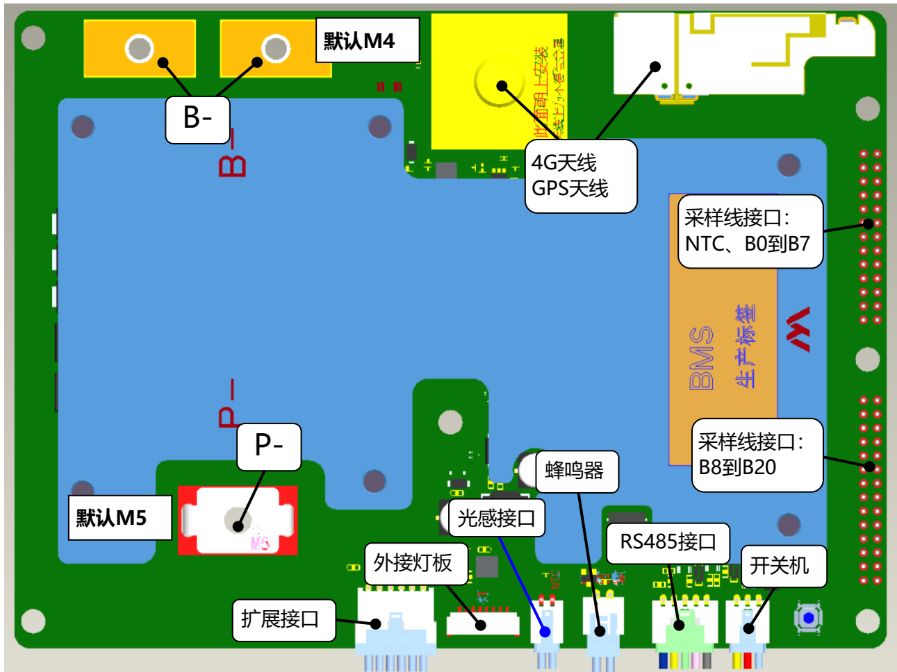
BM582接插件详细型号说明
