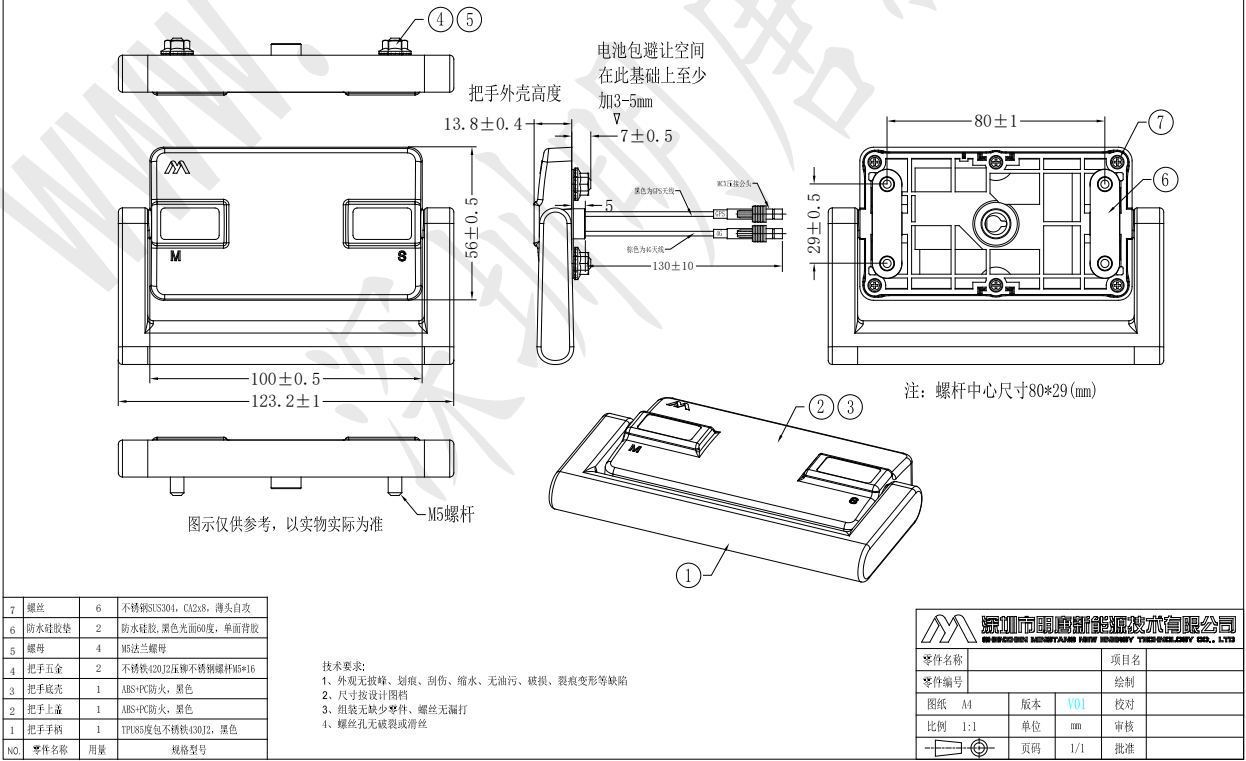
BM103-天线把手图档
