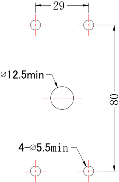
把手开孔尺寸参考图
