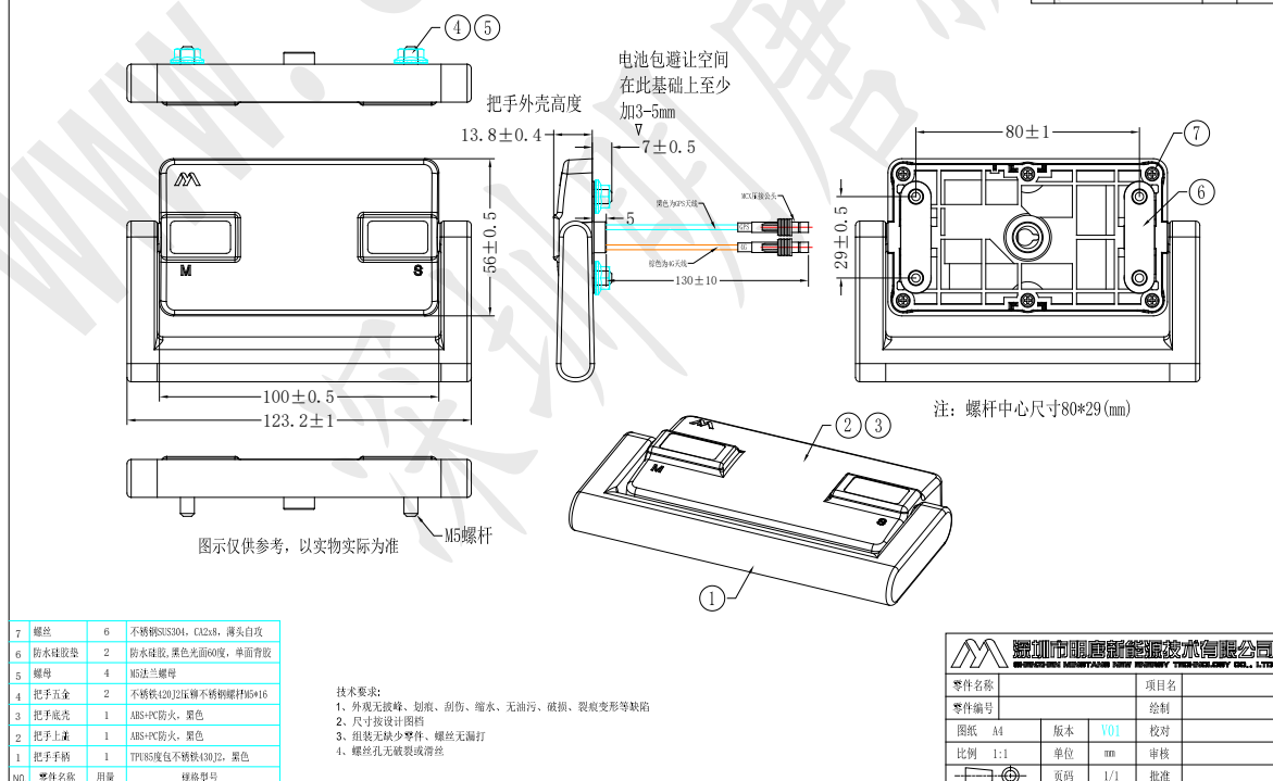
BM103-天线把手图档
