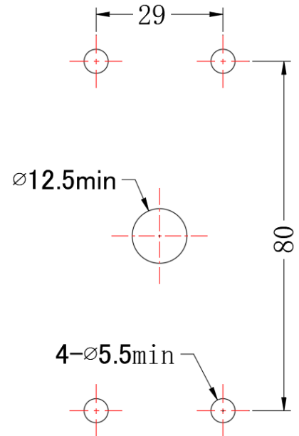
把手开孔尺寸参考图
