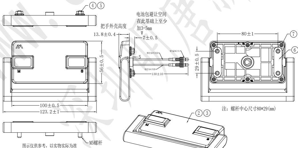
BM103-天线把手图档
