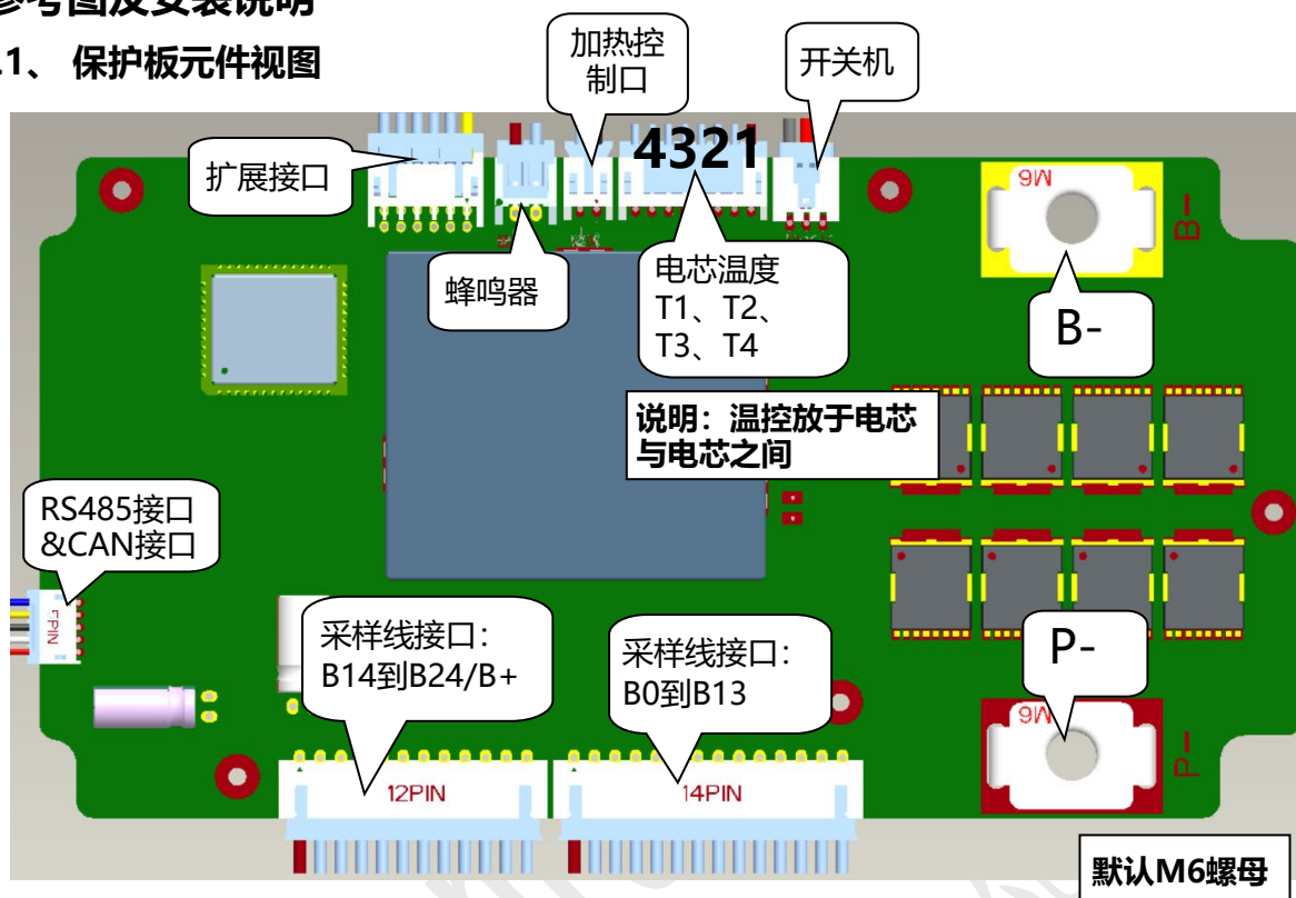
BM569K接插件详细型号说明
